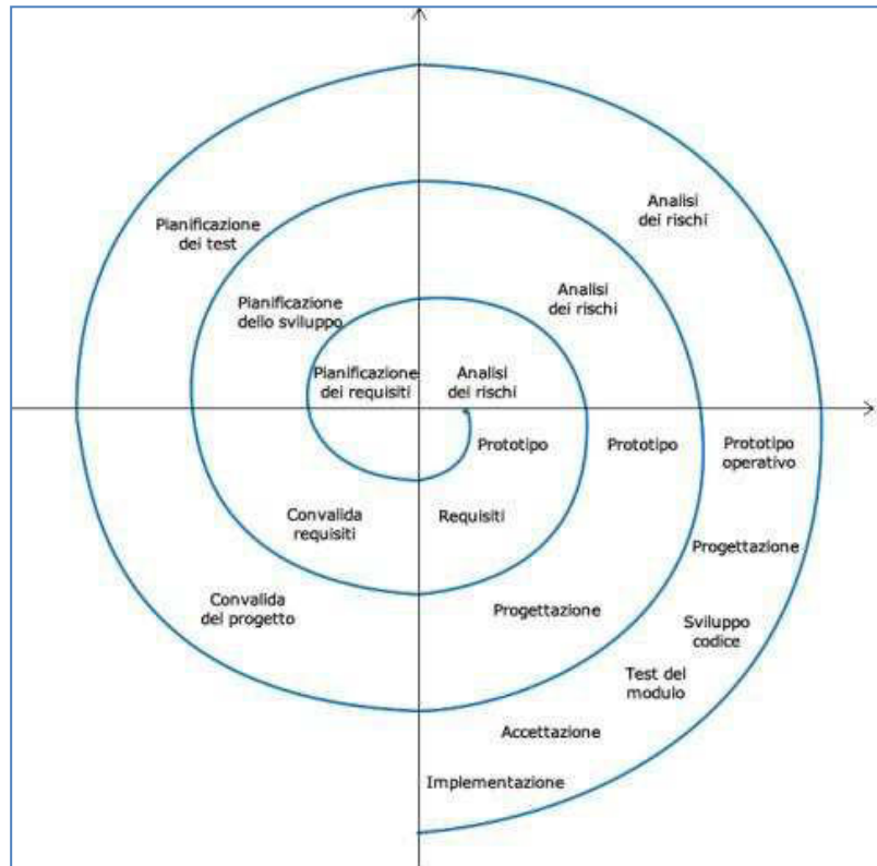
Figura 55: modello a spirale di sviluppo del software
